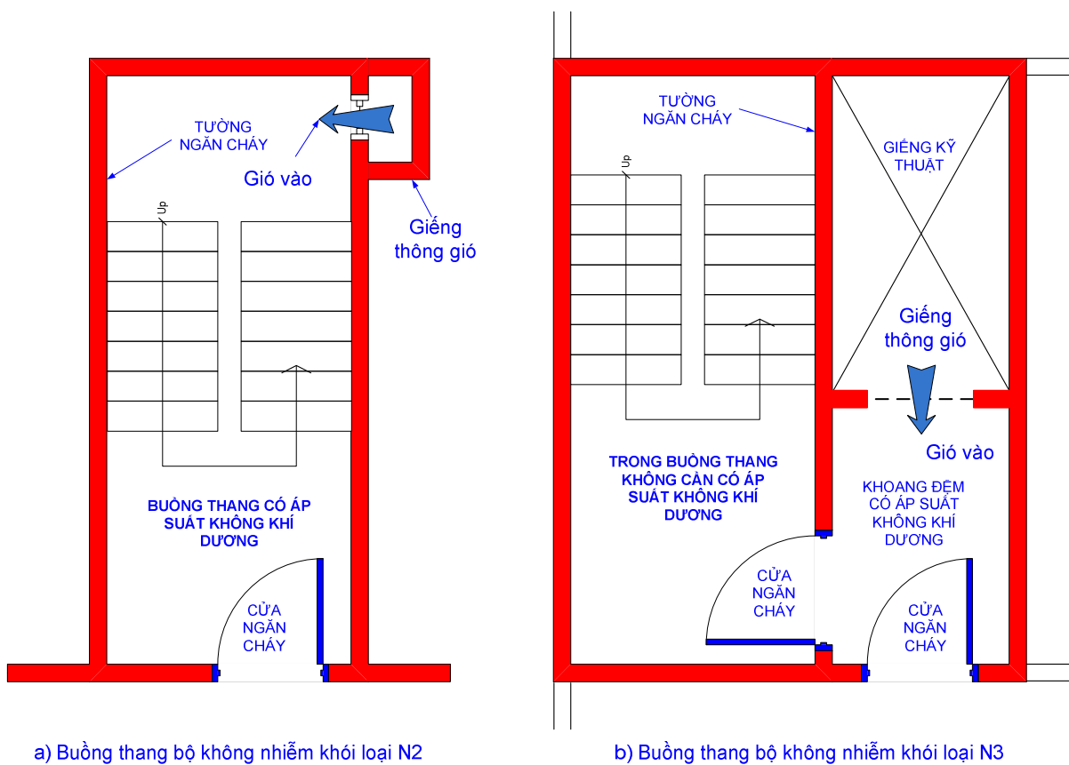
Hình I. 4 - Ví dụ minh họa buồng thang bộ không nhiễm khói loại N2 và N3
